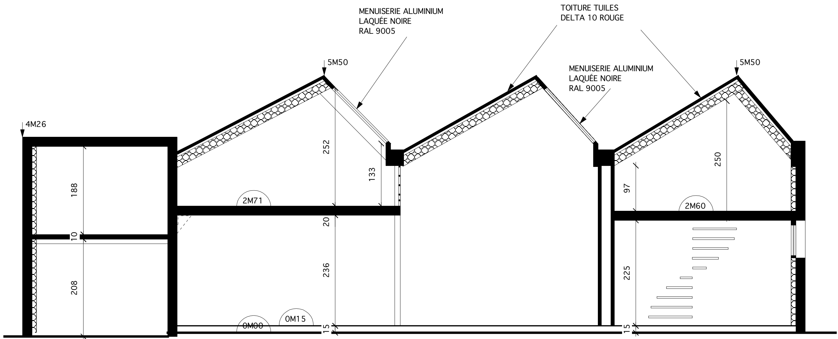
PROJET COUPE AA ECH: 1/50E
